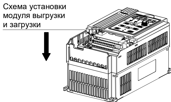
Рисунок В-2. Установка модуля выгрузки и загрузки
