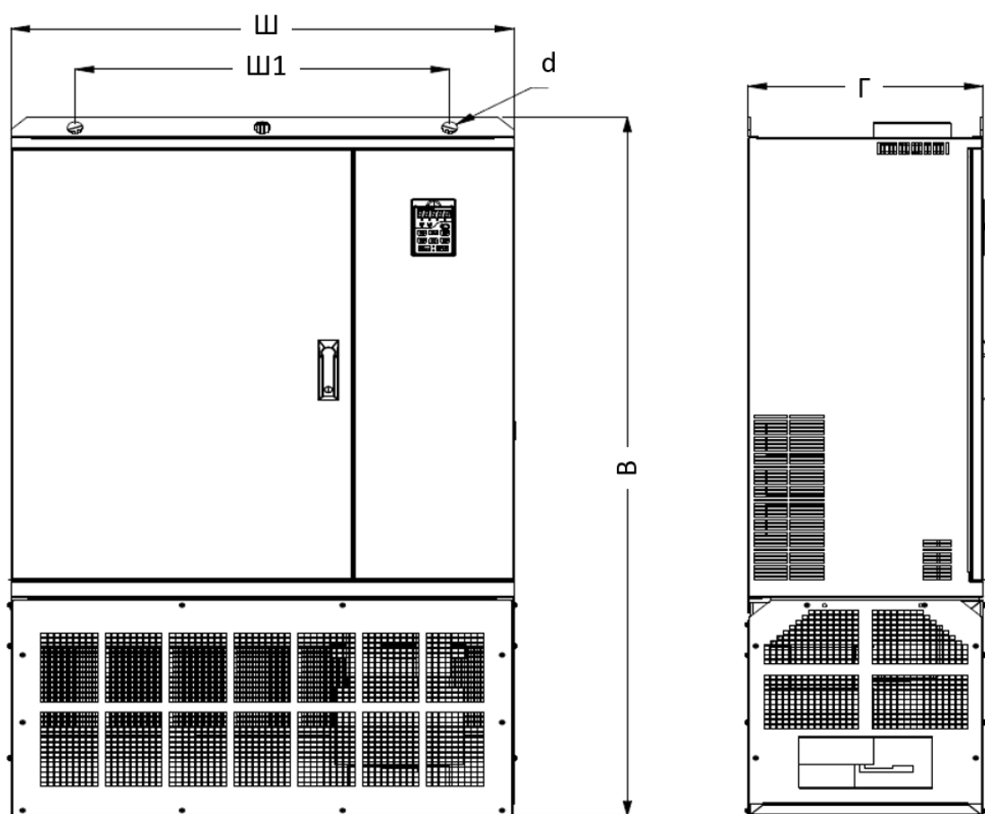
Рис. 2-9. ПЧ 450 - 630 кВт
