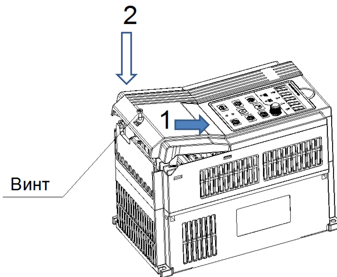
Рис. 3-7(e). Монтаж кожуха
