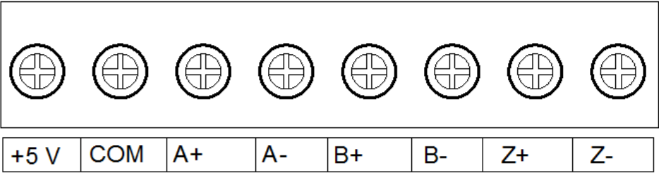
Рис.3 EXC-PG01 клеммник
