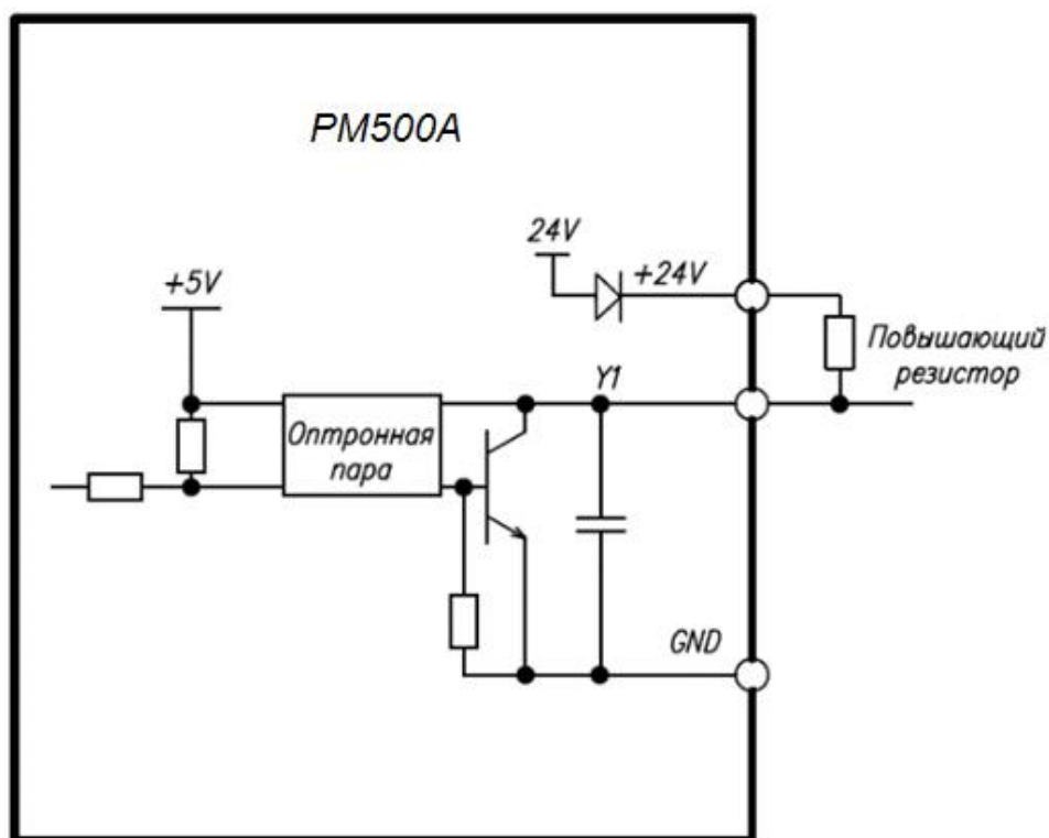
(a) Внутренний источник питания
