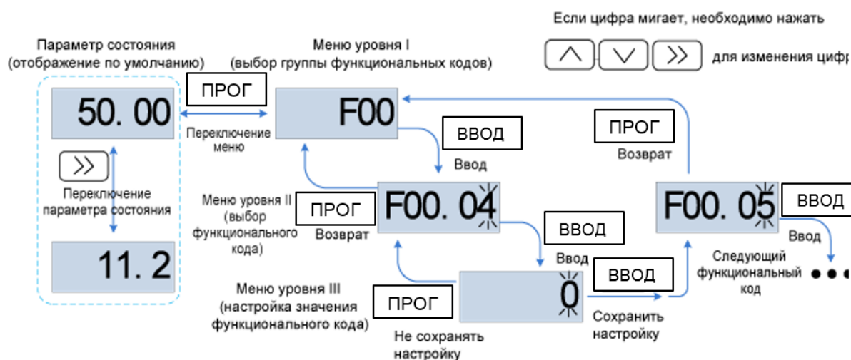
Рис. 4-2. Схема работы с панелью управления
