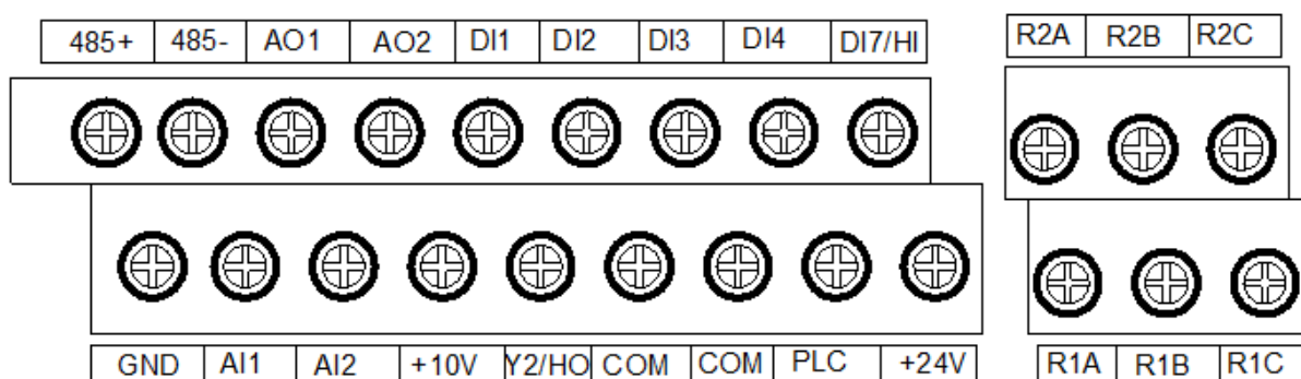
Рис. 3-17а. Клеммы цепи управления, модели РМ500А и РМ500Е до 2,2 кВт включительно
