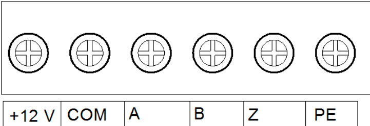
Рис.4 EXC-PG02 клеммник
