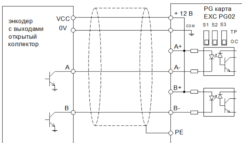
Рис. 5-5 Принципиальная схема подключения EXC-PG02 и энкодера с выходами открытый коллектор
