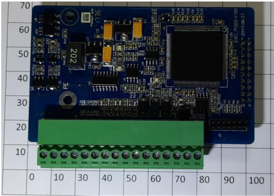
Рис.9 EXC-PG05B ECU1313 PG клеммы. Плата для ПЧ 4,0 и 5,5 кВт и выше
